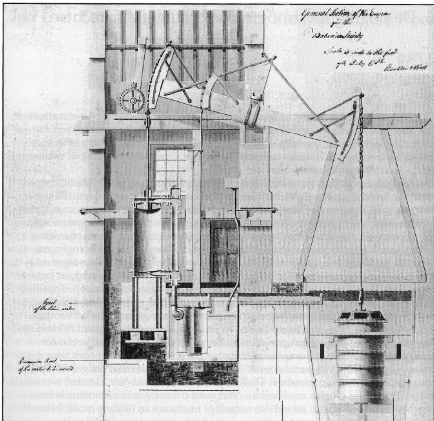
Het stoomgemaal van de polder Blijdorp zoals in 1786 getekend door Boulton & Watt, de leveranciers van de stoommachine.
