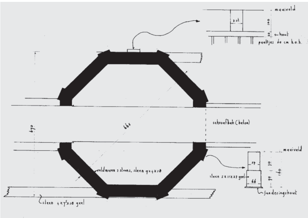
Opmetingstekening van de funderingsresten van de Aylvamoelen.
