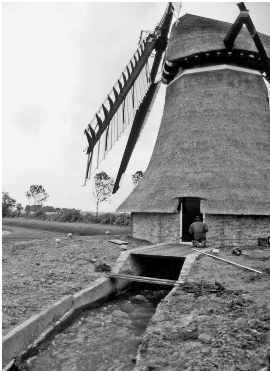
Op 23 mei 2000 werd het eerste water met de verplaatste molen uitgemalen. Let op de gebogen voorwaterloop of uitschoot.
